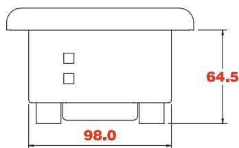
< 하측면도 >
