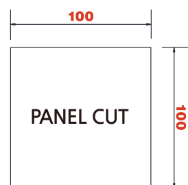
< PANEL 타공도 >
