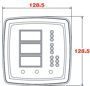
< 정면도 >
