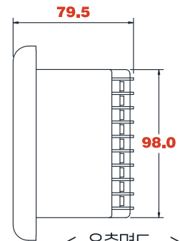
< 우측면도 >
